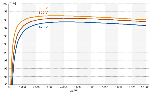
Courbes caractéristiques du rendement de blueplanet 10.0 TL3
